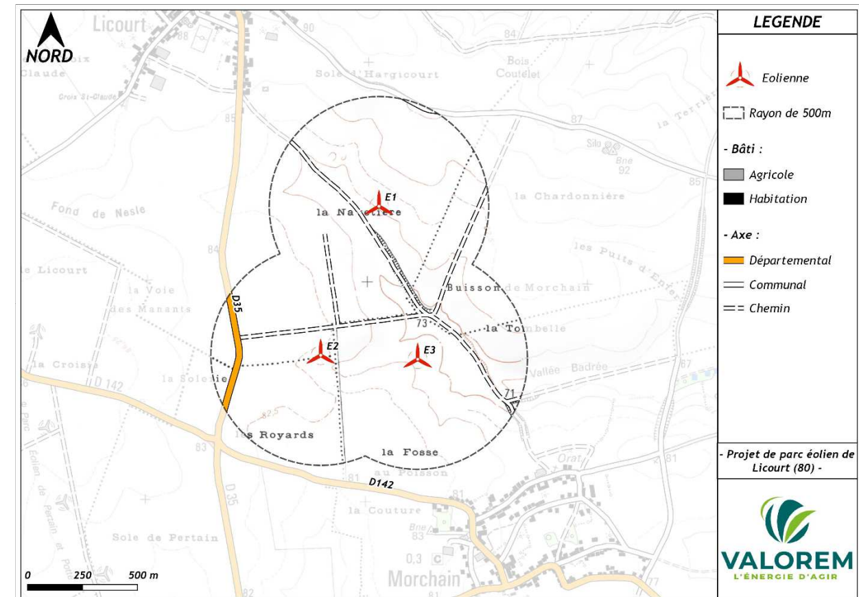
Aire d'étude de l'étude de dangers du parc éolien de Licourt
