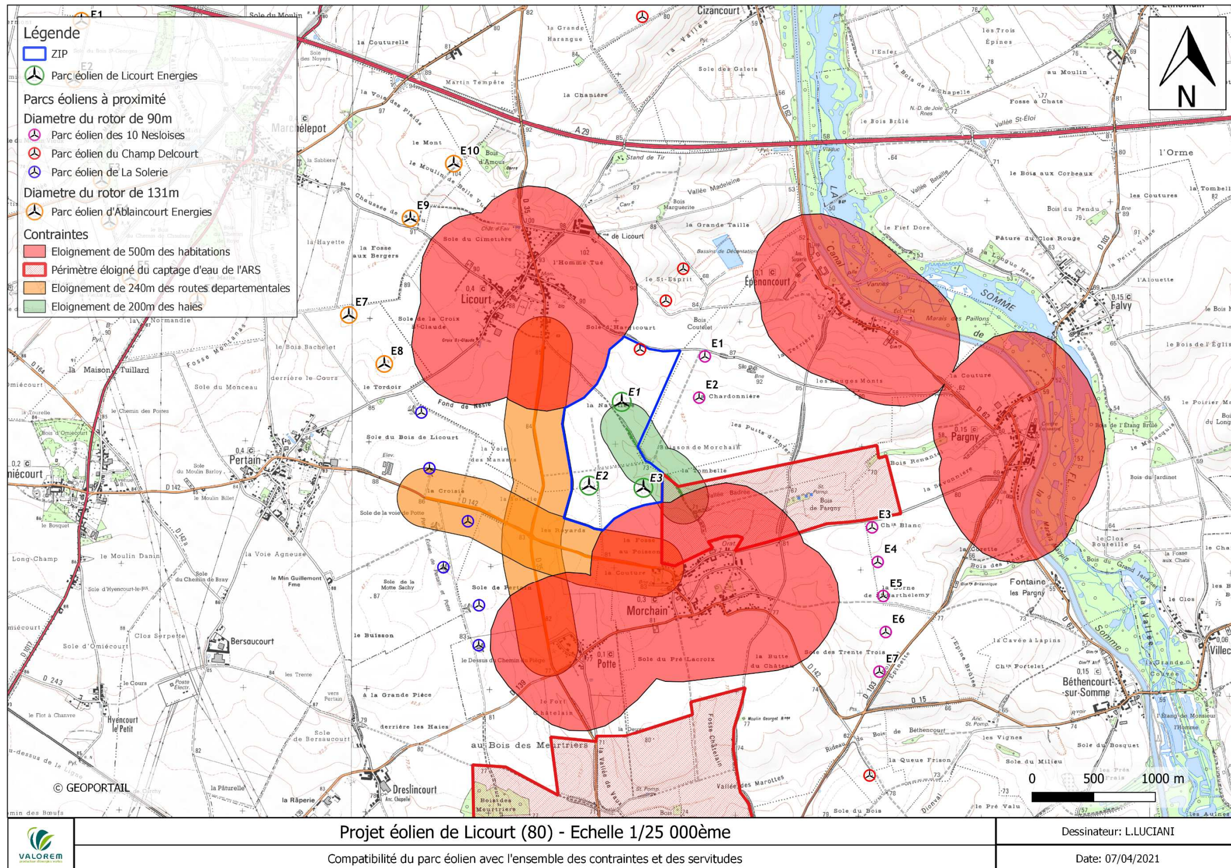
Cartographie des principales contraintes liées aux servitudes
